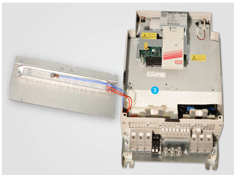
2. Sovitish ventilyatorlarni almashtirish uchun modulli korpus
